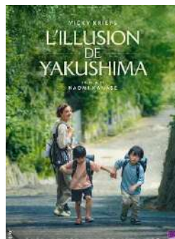
L'illusion de Yakushima
